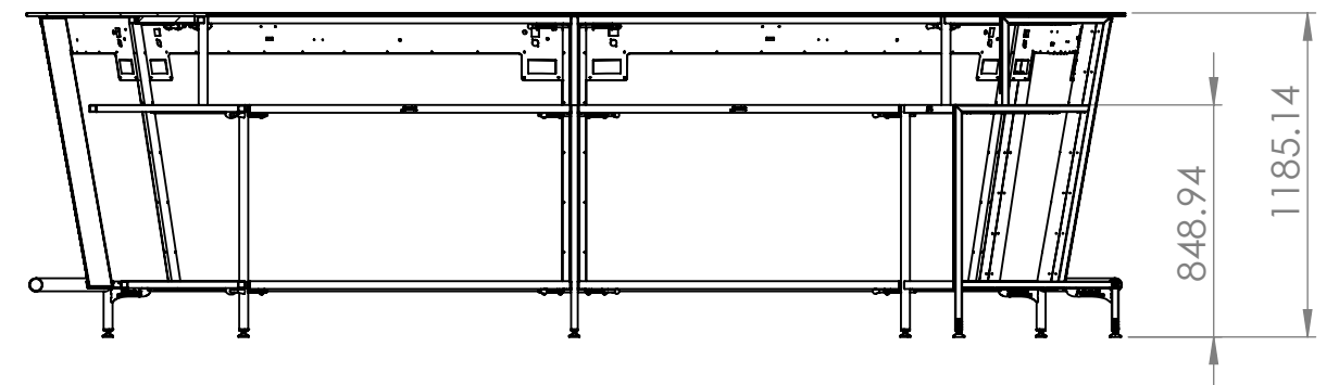
SECTION A-A SCALE 1 : 30
